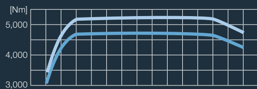
Torque V12-1400 / V12-1550
